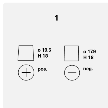
Typ biegunów
