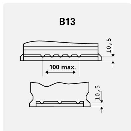
Docisk podstawy
